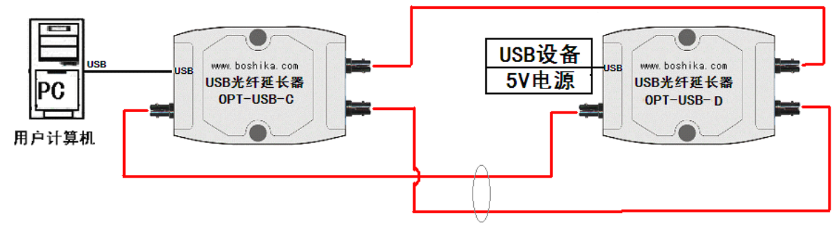
图 2 OPT-USB 的典型应用
