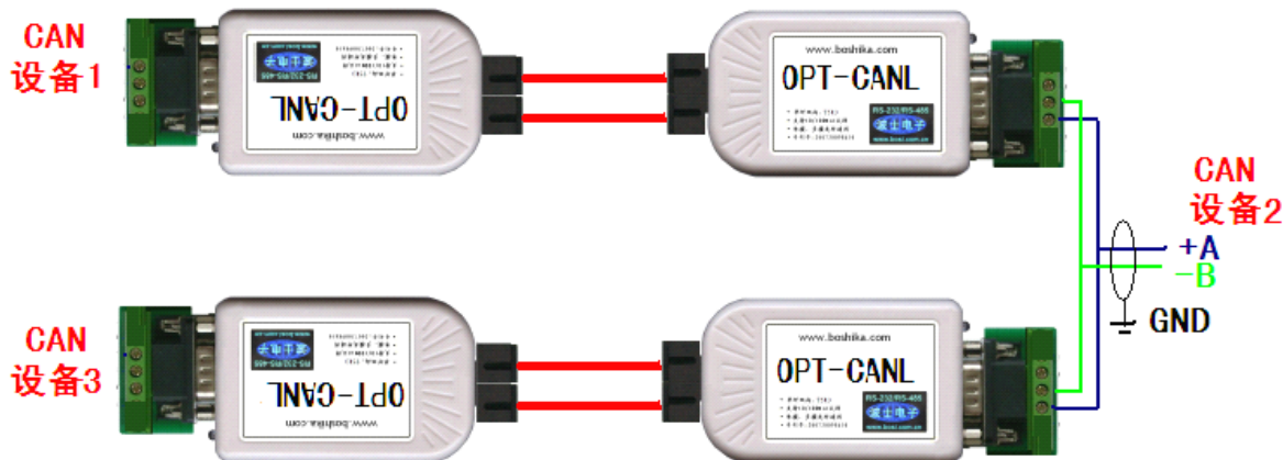
图 3 双纤多机通信
