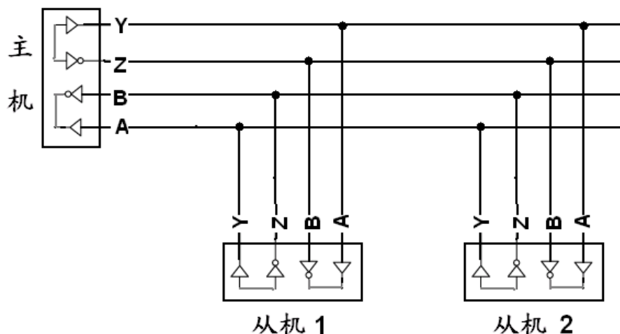
图4 典型的全双工多机通信图
